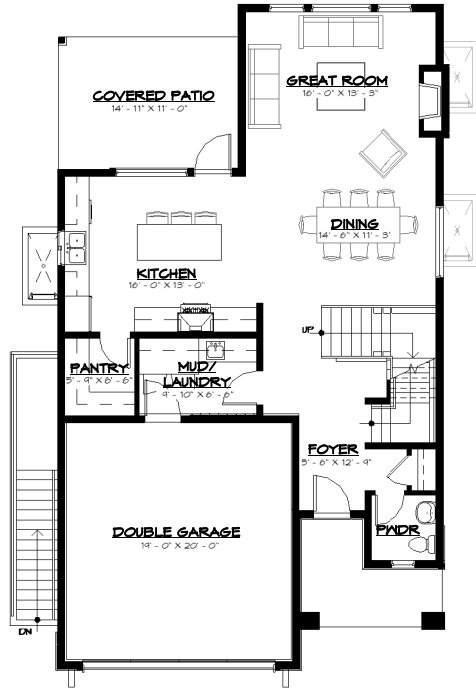
MAIN FLOOR PLAN - E1
