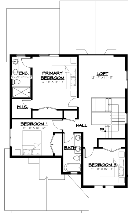
UPPER FLOOR PLAN - E1
