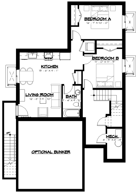
BASEMENT FLOOR PLAN - E1
