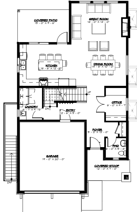
MAIN FLOOR PLAN - D1
