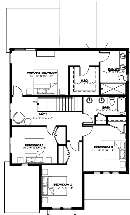
UPPER FLOOR PLAN - D1
